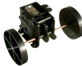
Moteur à courant continu Avec réducteur de vitesse par engrenage plastique 4 € l'unité
